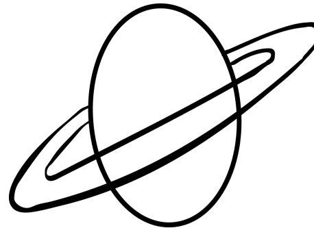
Saturno
